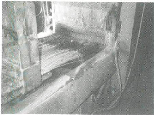
Zelf ontworpen en geconstrueerde teensnijmachine.
