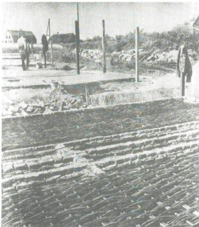
Wilgenvloermatten een "Staaltje" van noodbewapening.
