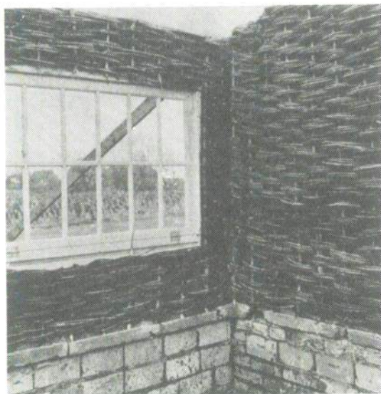
Detail van hoek, raam en trasraamaansluitingen.
