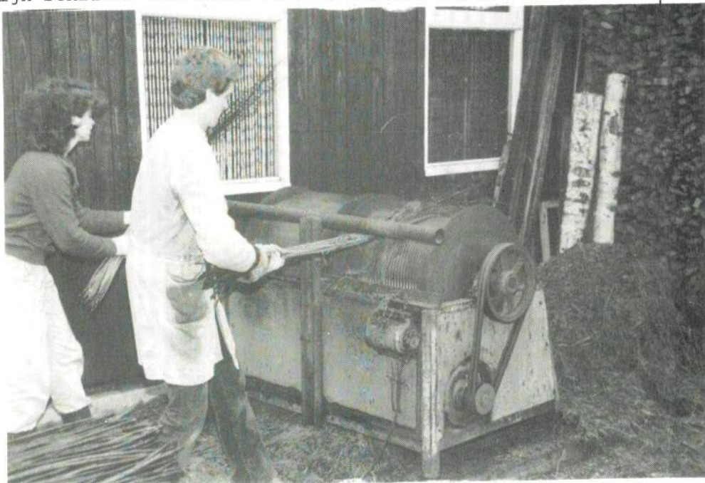
Het schillen van buffteen met de schilmachine door amateur en vakman (Kooijmans jr.)
